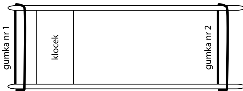
Konstrukcja pierwszego i ostatniego modułu
